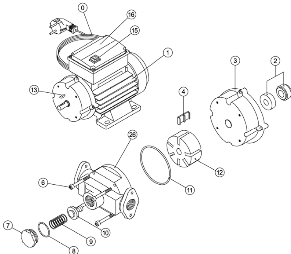
SAG-88 0,37kW SEM BASE METÁLICA Peso: 15,05Kg Tamanho: 450x320x190mm
