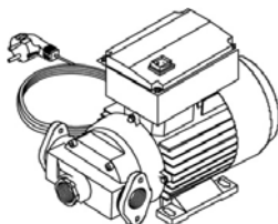
AG-88 0,37kW Peso: 13Kg Tamanho: 310x165x205mm
